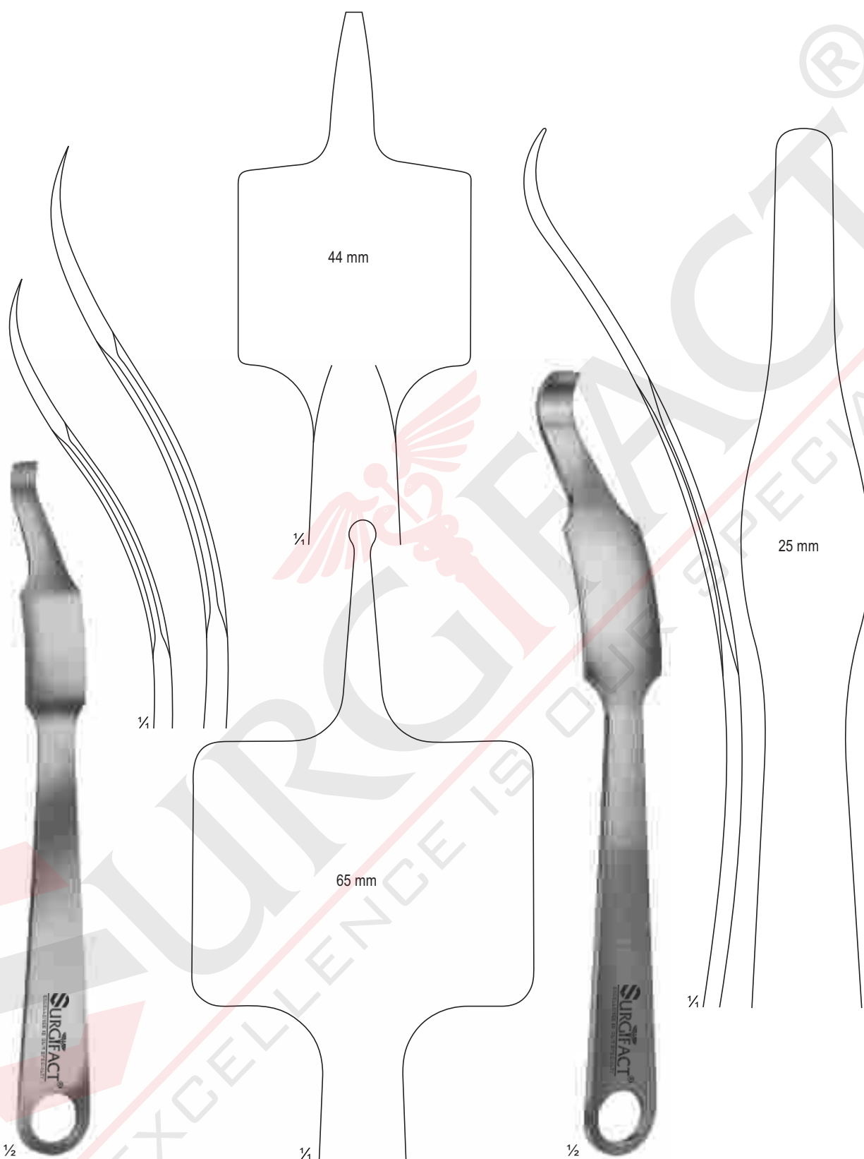
SF-20-018 - 019 VERBRUGGE-MULLER SF-20-018 240 mm SF-20-019 255 mm
